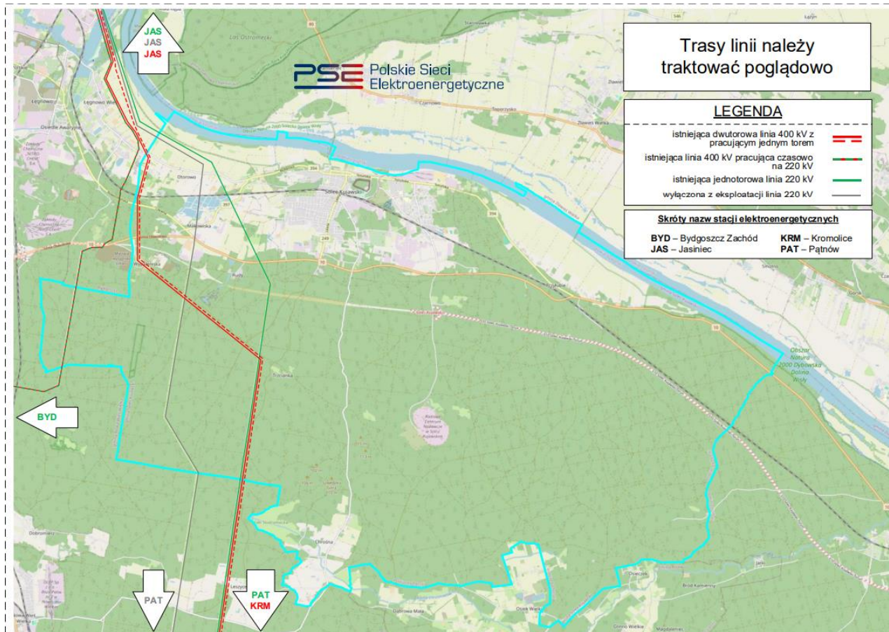
Mapa 8. Schemat KSE na terenie Gminy Solec Kujawski
